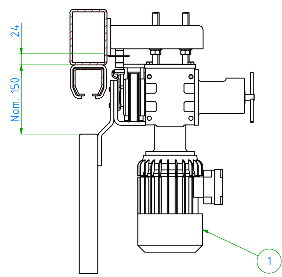
A-A (1:5)
